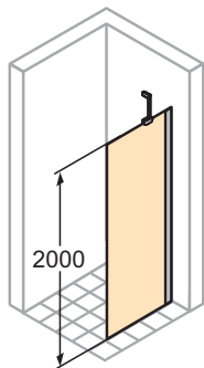
Upevnění vpravo
